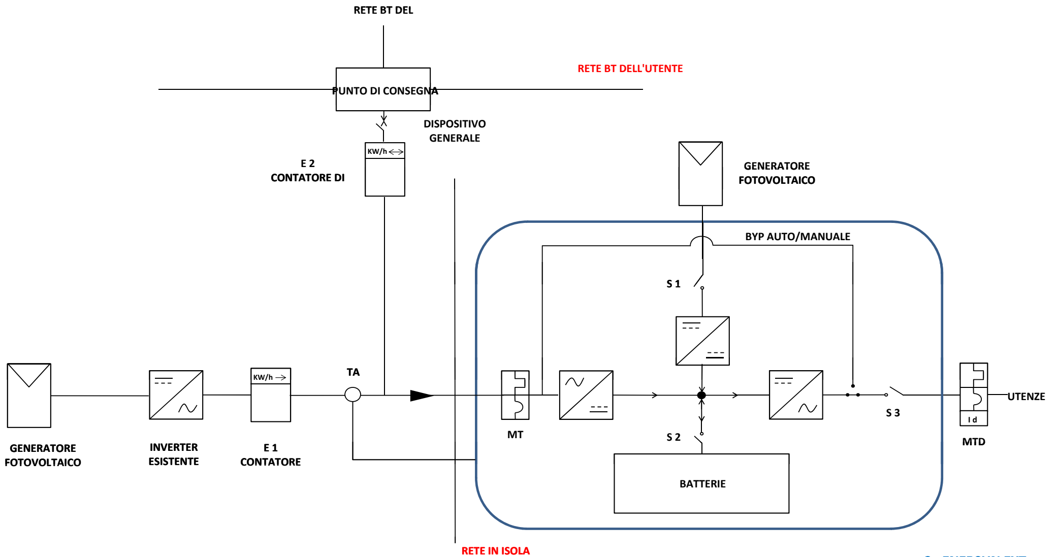
3. ENERSUN EXT Impianti esistenti con ampliamento
